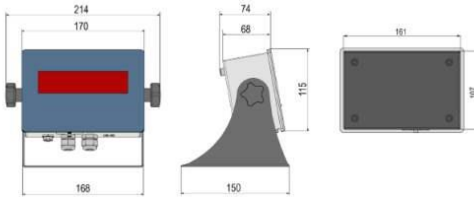
Afmetingen van het display van massa weegstelsel / silo weegschaal van de KCPN-DGT 20 serie
